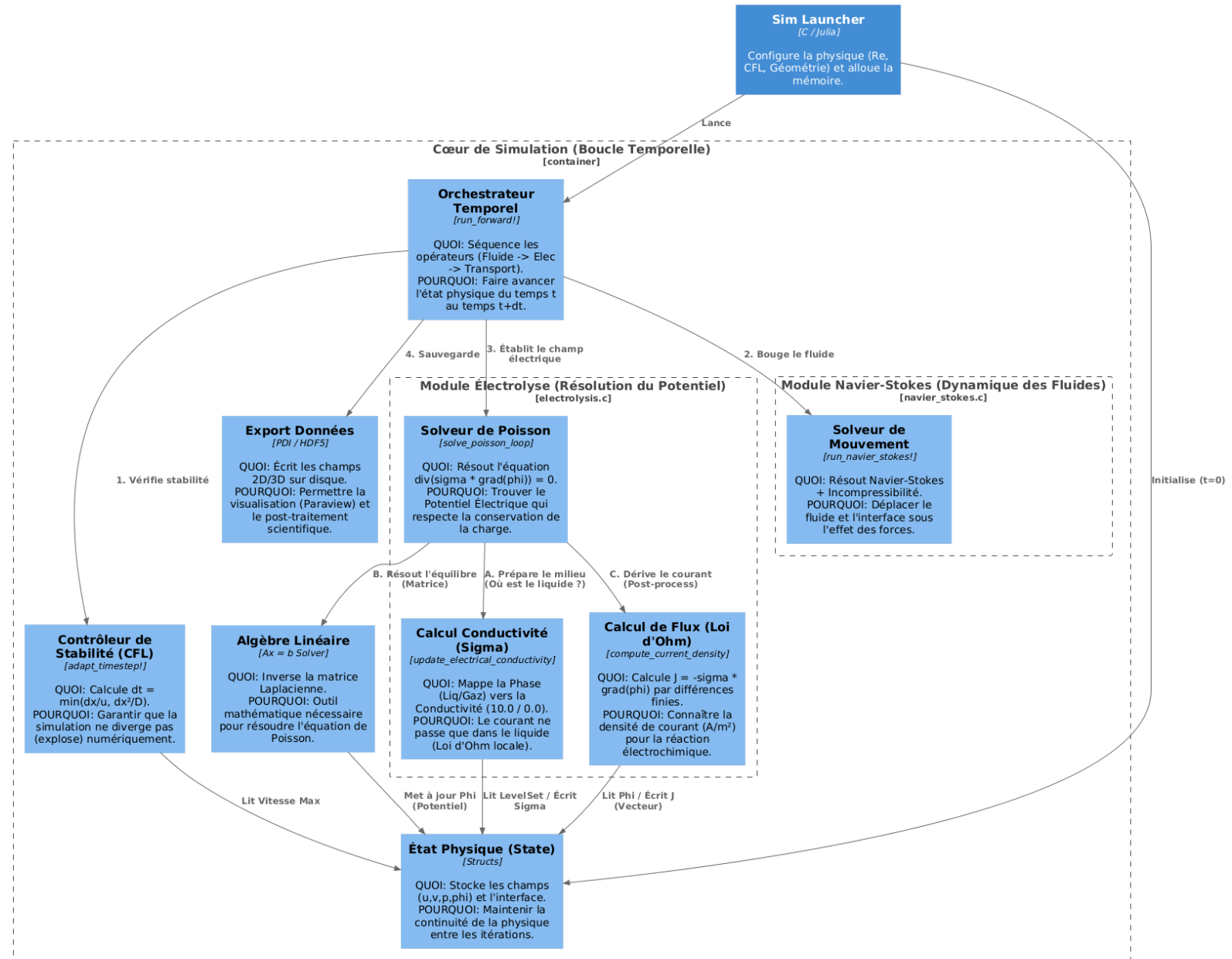
Diagramme C4 (Niveau 3) - Logique Fonctionnelle & Physique
