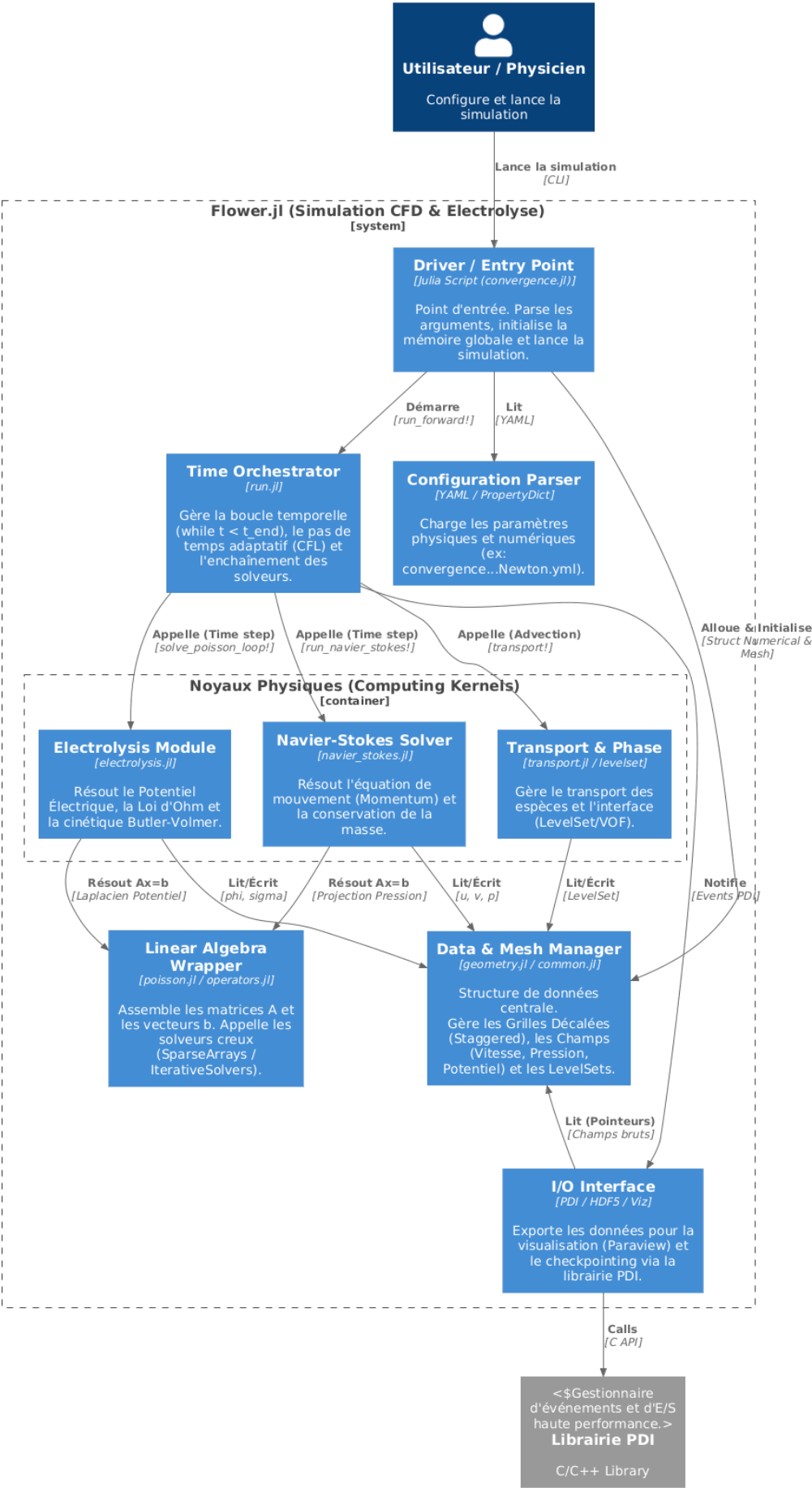
Diagramme C4 Container - Architecture Actuelle de Flower.jl
